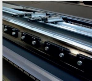
Europen Type V Die Holder
